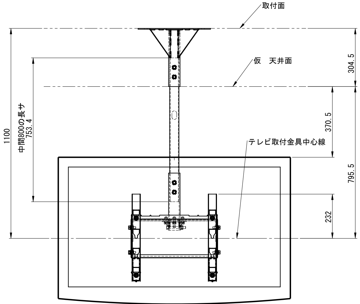
Panasonicビエラ TH-P50G2 PAF04RU+ATC-UP800組合せ例
