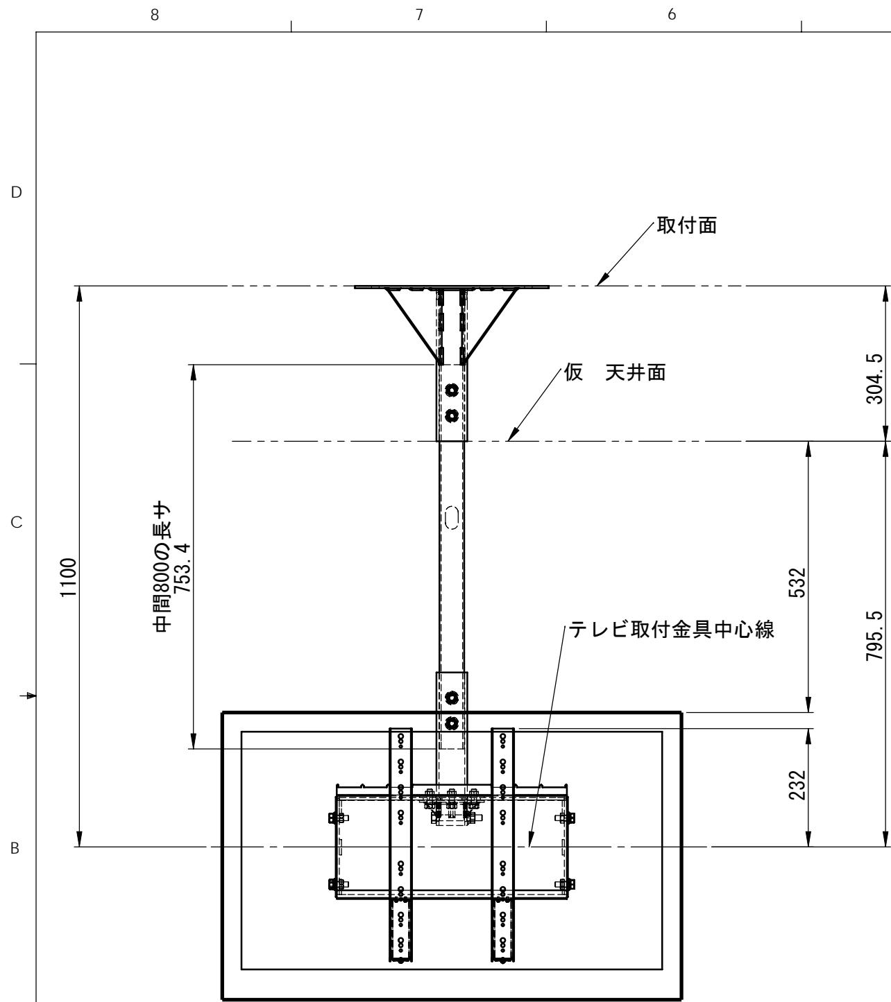
三菱REAL LCD-37MXW100 ATC01RU+ATC-UP800組合せ例
