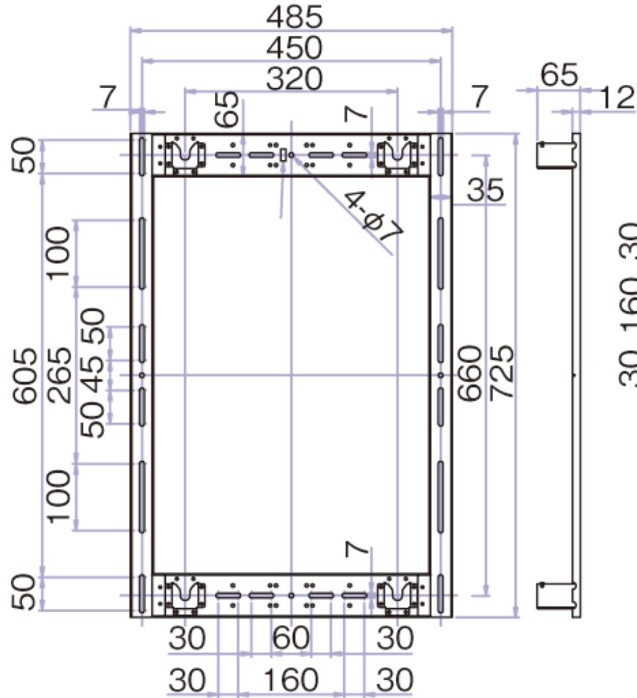
縦取付寸法
