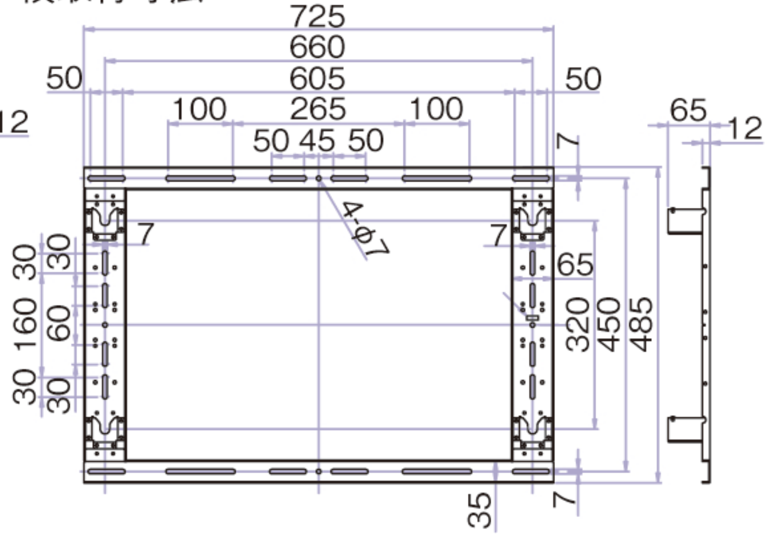
横取付寸法
