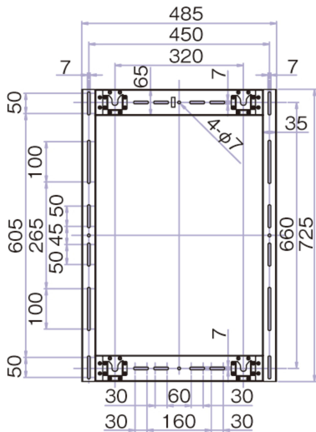
縦取付寸法
