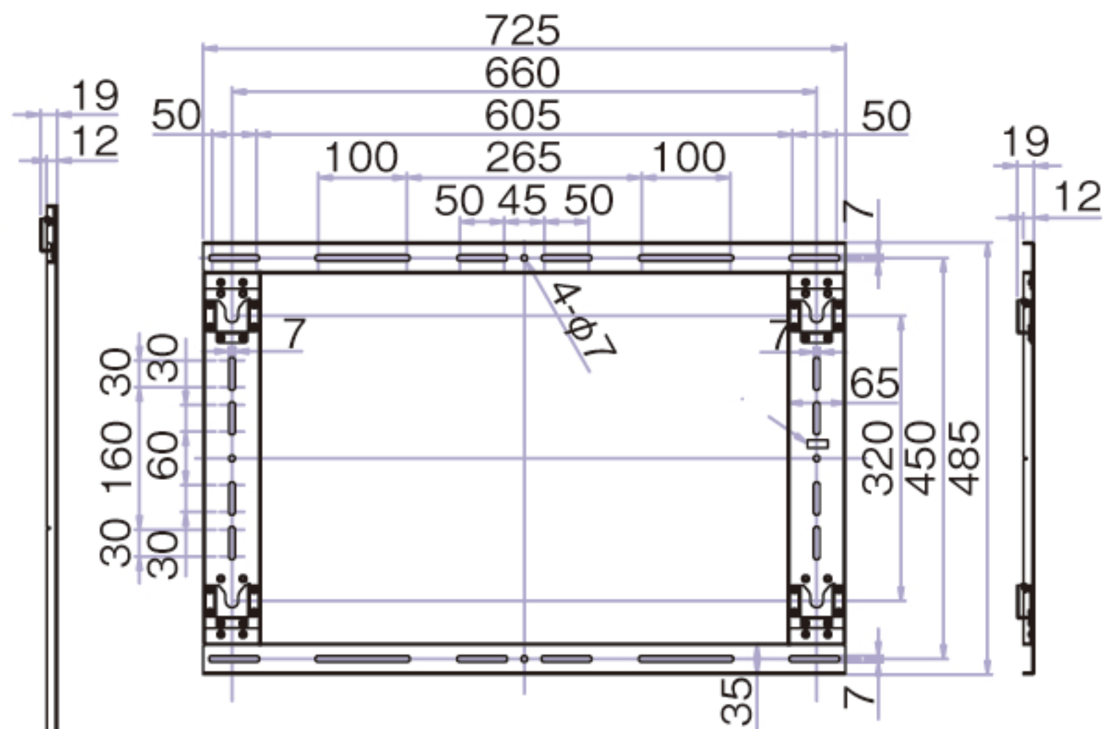
横取付寸法
