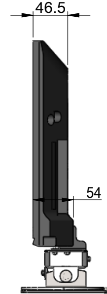
チルト可動範囲
